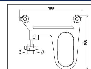
PENDANT TROLLEY MCRT12
